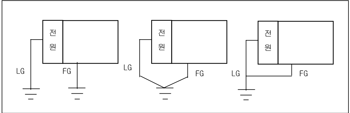
가) 전용접지 : 가장 좋음
